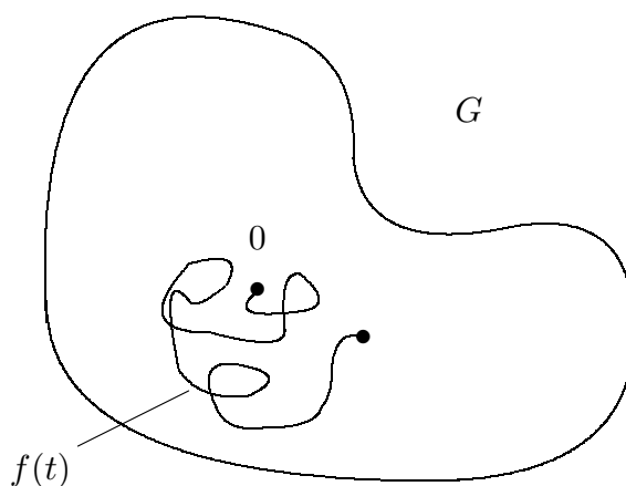
Trajektorien der Brownschen Bewegung
